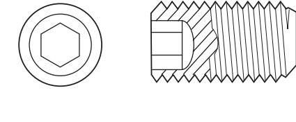
VIS D'ARRÊT SANS TÊTE À 6 PANS CREUX SOCKET SET SCREWS
