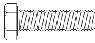
BOULONS À TÊTE HEXAGONALE À FILET COMPLET HEX HEAD CAP SCREWS FULL THREAD
