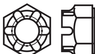
ÉCROUS À CRÊNEAUX DÉGAGÉS CASTLE NUTS
