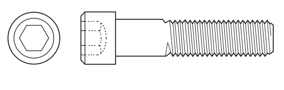
VIS CALIBRÉES À TÊTE CYLINDRIQUE À 6 PANS CREUX SOCKET CAP SCREWS
