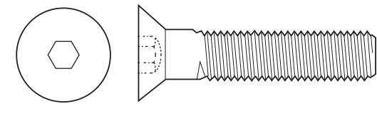
VIS CALIBRÉES À TÊTE PLATE À 6 PANS CREUX FLAT SOCKET CAP SCREWS
