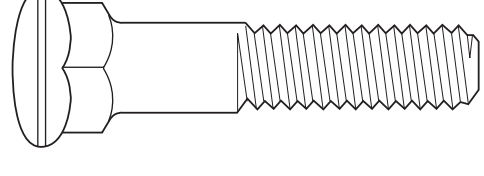
BOULONS DE NIVELEUSE À TÊTE CALOTTE DOME HEAD SCRAPER BLADE BOLTS
